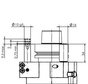
HSK - F63 Weinig
