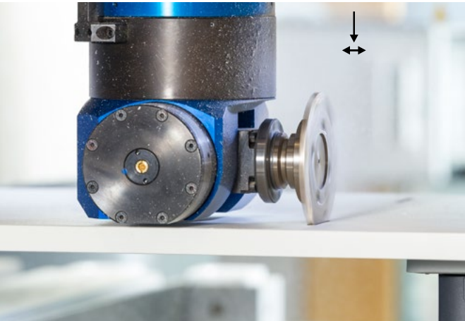
Fräsen der Profilnut zum Einsetzen des Verbinders am Gegenstück (vertikale Bearbeitung).
