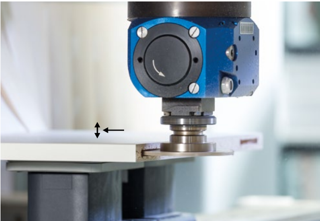
Fräsen der Profilnut zum Einsetzen des Verbinders (horizontale Bearbeitung).
