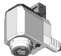
Radial-Bohr und Fräskopf, VDI 20, mit IK Radial drilling and milling head, VDI 20, with IC
